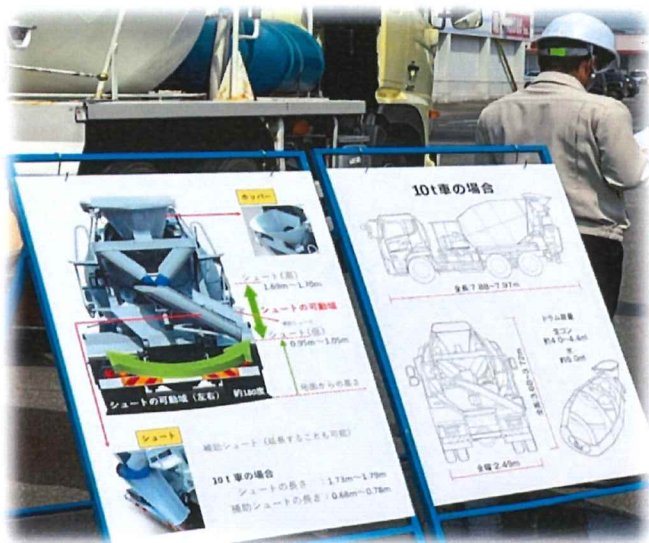
アジ車 構造説明パネル
